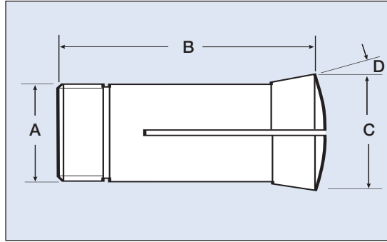
Dimensions
